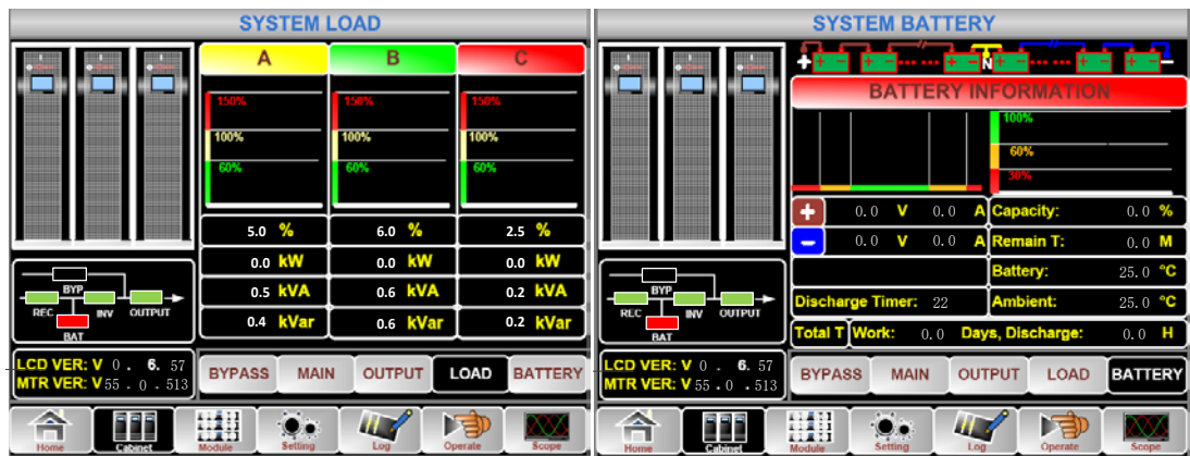
Рис.3-5Интерфейс подменю распределительного шкафа
