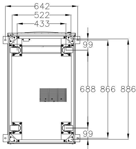
(а) Опорная конструкция для 60 кВА, 90 кВА и 120 кВА (Вид снизу, единицы измерения: мм)
