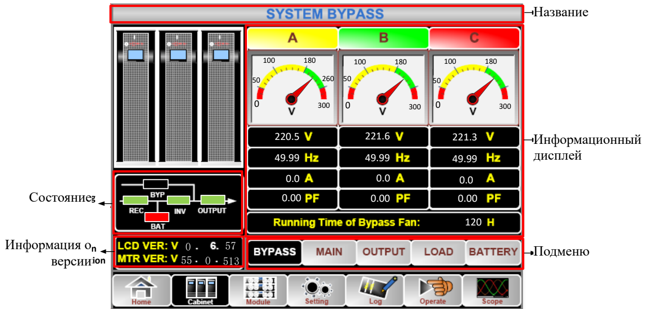
Рис.3-4 Шкаф
